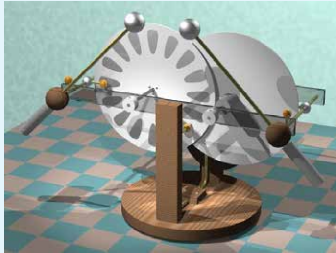
Fig. 1. Máquina Wimshurst
