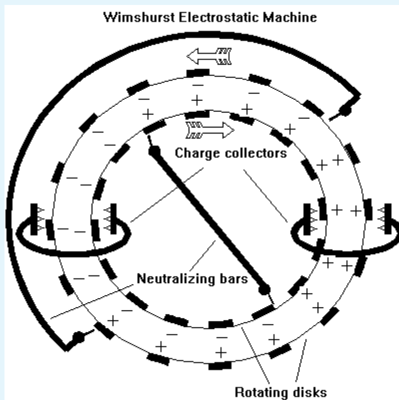
Fig. 2. Esquema de funcionamiento de la maquina Wimshurst.
