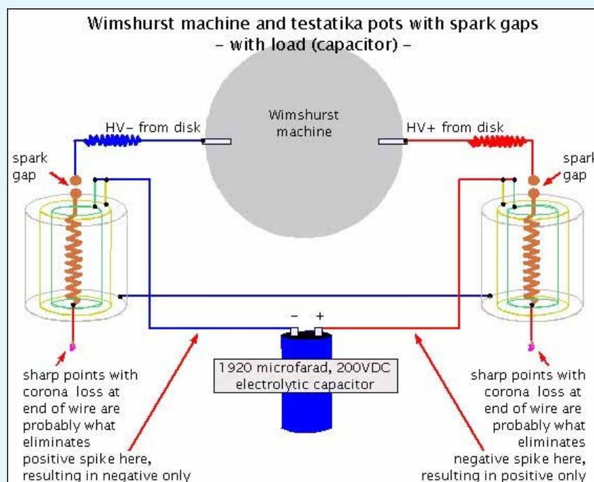
Fig. 3. Máquina Testarika.
